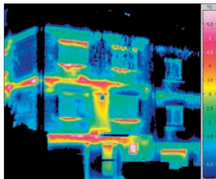
Thermographieaufnahmen – die Farbleiste rechts am unteren Bild macht deutlich, wie wichtig Dämmung ist.
